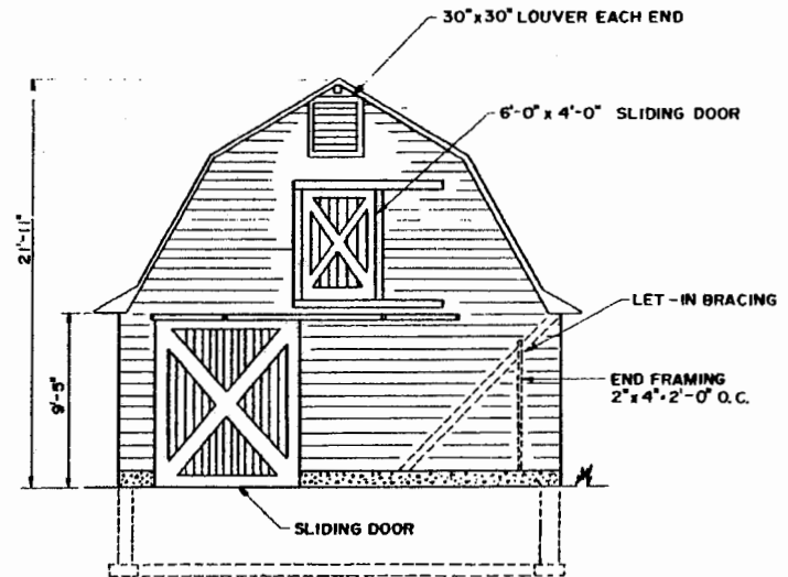
END ELEVATION
