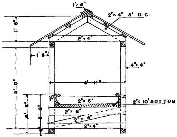
END ELEVATION
