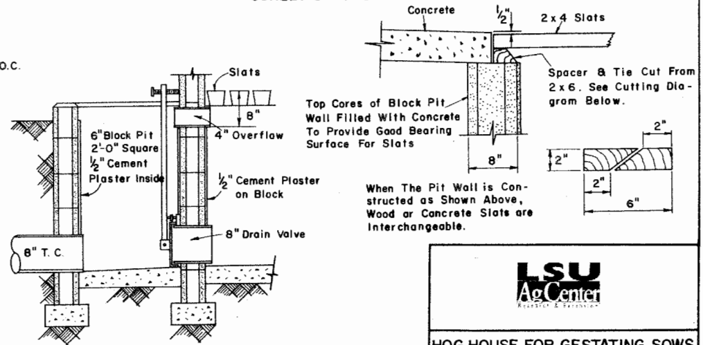
Section "B-B" SCALE: \frac{3}{4}'' = 1'-0''
