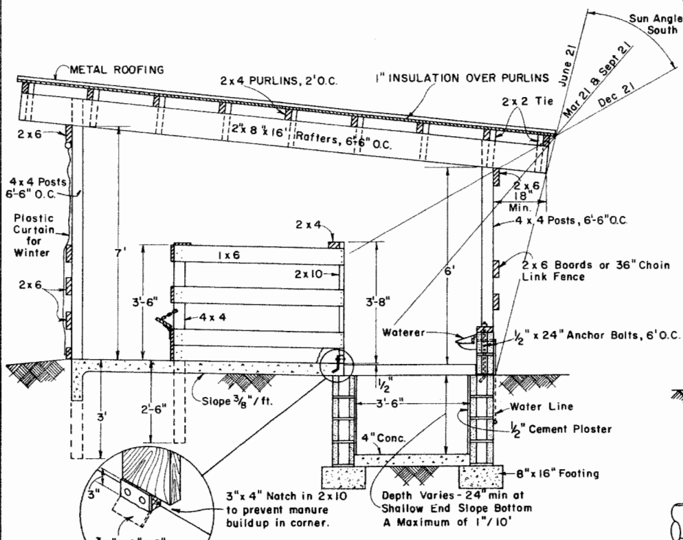
Section "A-A" SCALE: \frac{1}{2}'' = 1'-0''
