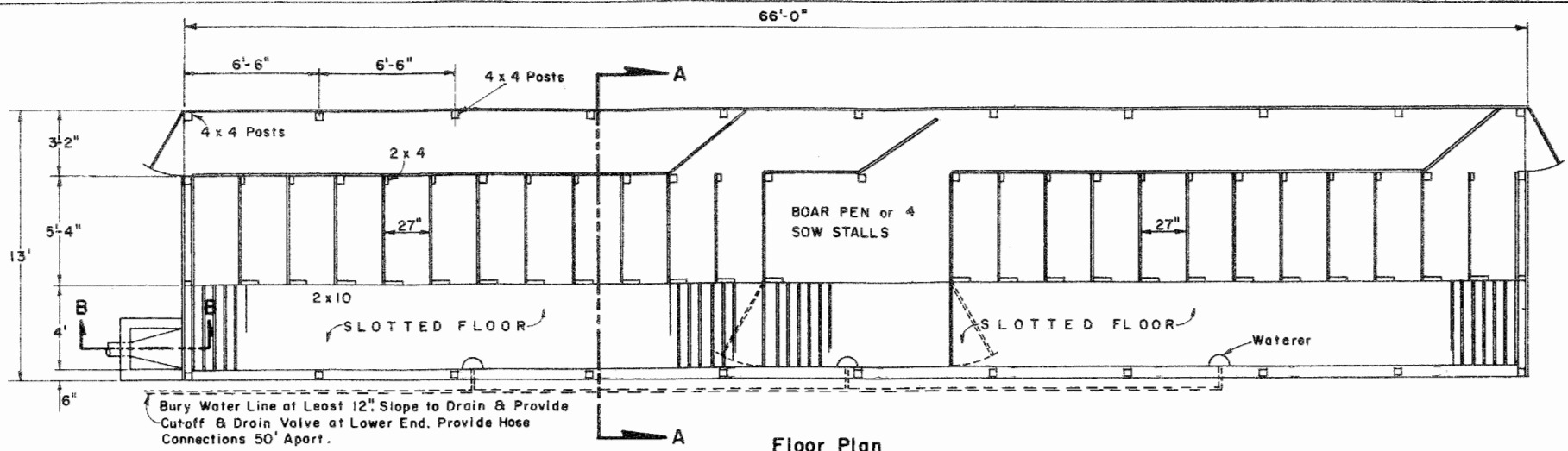
Floor Plan SCALE: \frac{1}{4}'' = 1'-0''
