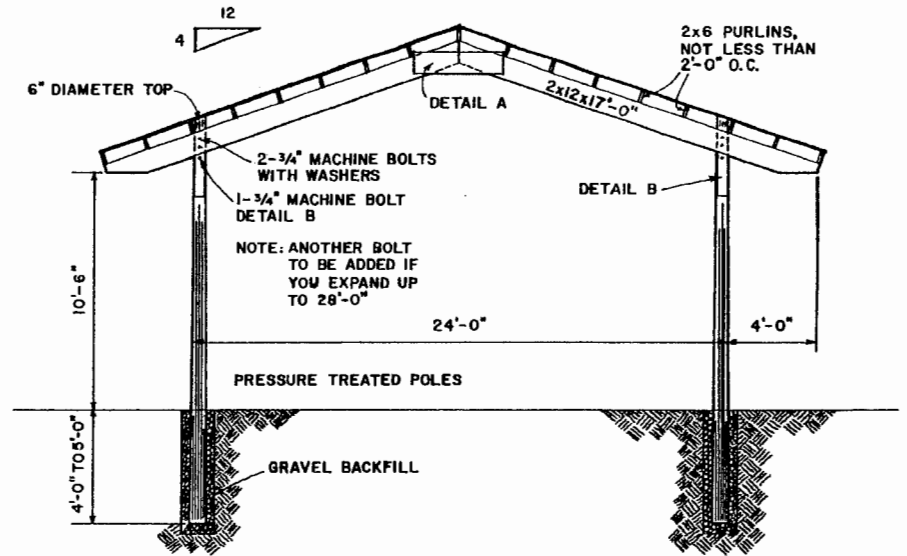
SECTION SCALE: 1/4"=1'-0"
