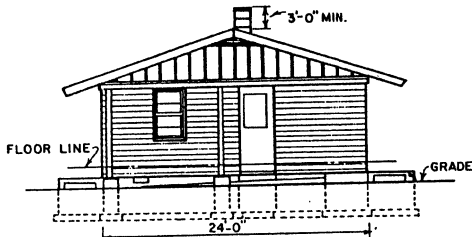
RIGHT ELEVATION
