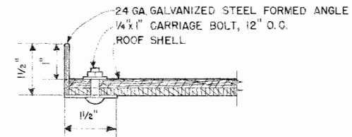
SECTION B-B SCALE: 6" = 1'-0"
