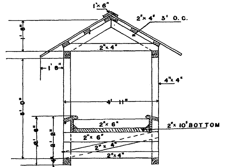
END ELEVATION
